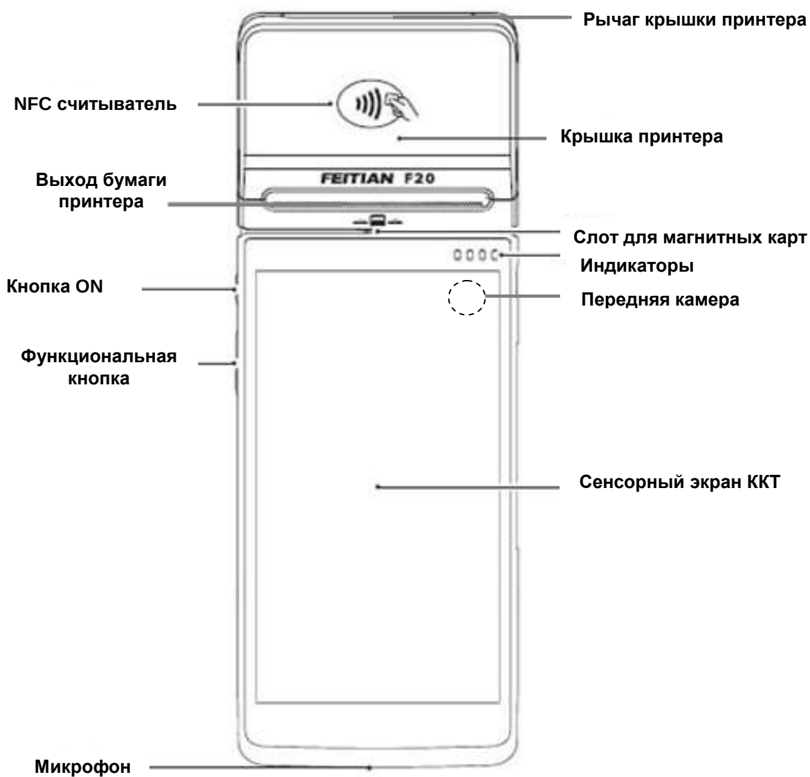
Рис 1. ККТ с модулем эквайринга (вид спереди)
